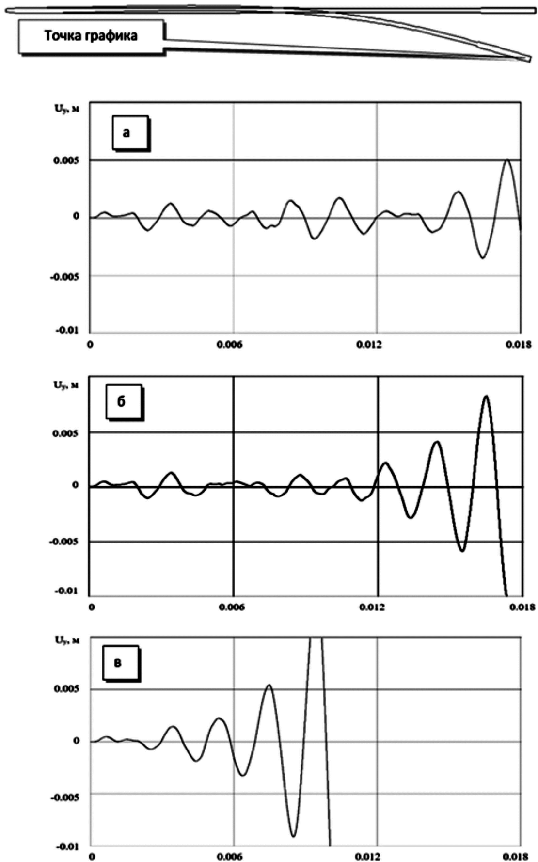
Рис.3. Графики перемещений концевой кромки пластины во времени при различных условиях аэродинамического нагрева (а – без изменения температуры, б – с теплозащитой поверхностей пластины, в – без теплозащиты)
