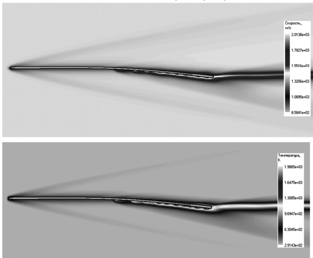
Рис. 2. Картина обтекания без угла атаки пластины потоком воздуха
